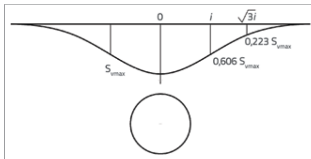
Slika 1. Poprečni profil slijeganja površine terena uslijed izgradnje tunela (Gaussova krivulja)
