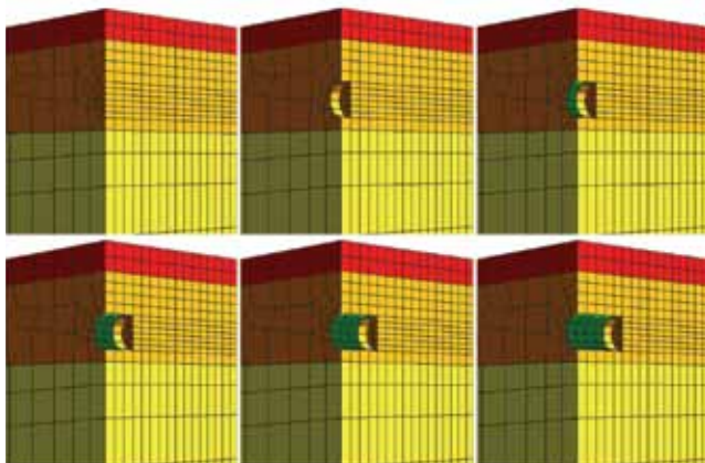
Slika 3. Sekvence 3D simulacije procesa izgradnje tunela
