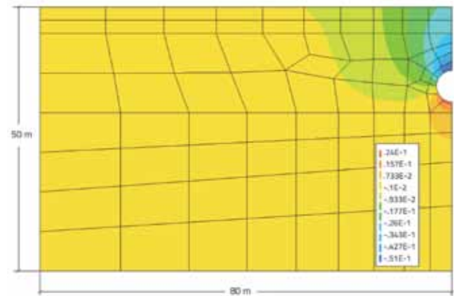
Slika 7. Konture vertikalnih pomaka u poprečnom presjeku y = -50 m
